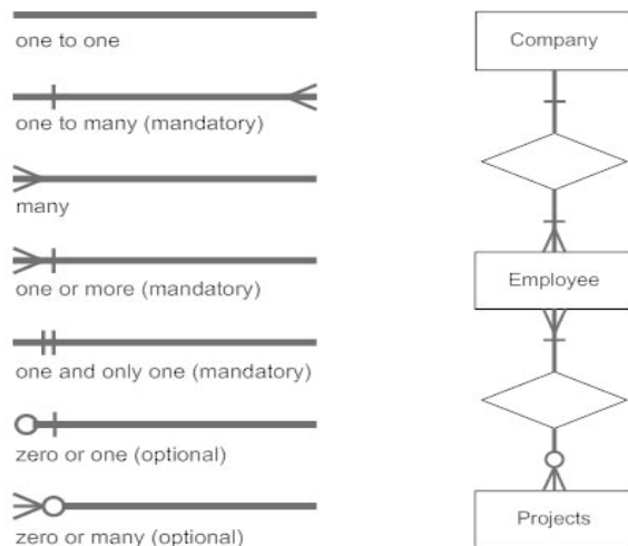
Fig: Notations of ER diagram
